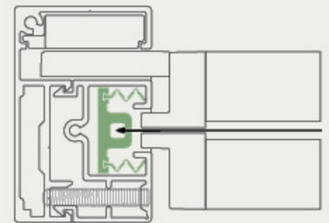
Detailansicht Zip / détail Zip
